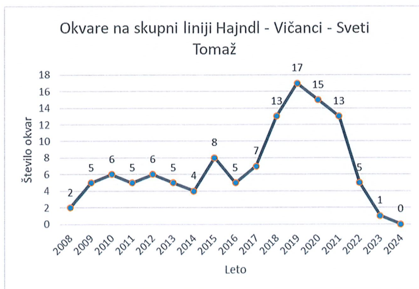
Slika 11: Prikaz okvar na Javnem vodovodnem omrežju na skupni liniji Hajndl – Vičanci - Sv. Tomaž
