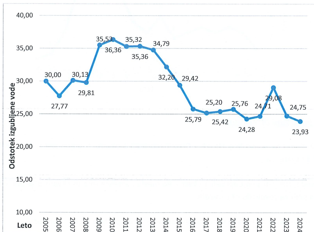
Slika 13: Gibanje izgubljene vode iz Javnega vodovodnega omrežja Ormož
